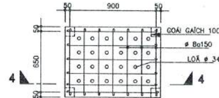
ĐÀN NGĂN LỌC H1 R.C PLATE H1
