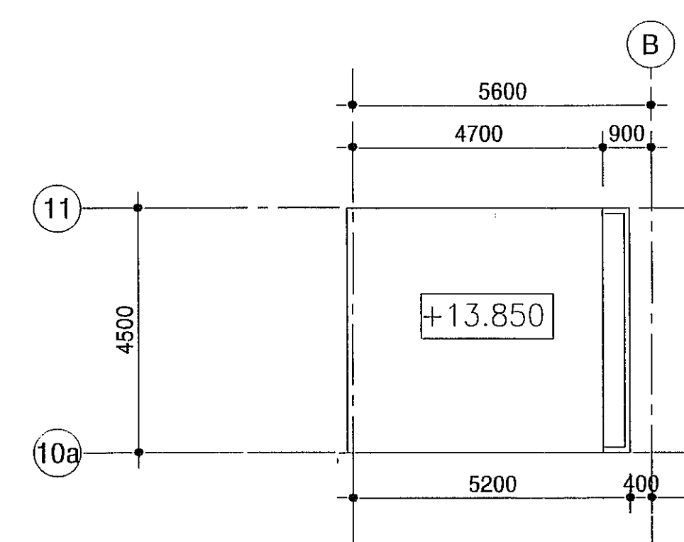
MẶT BẰNG MÁI THANG MÁY(+13.850)
