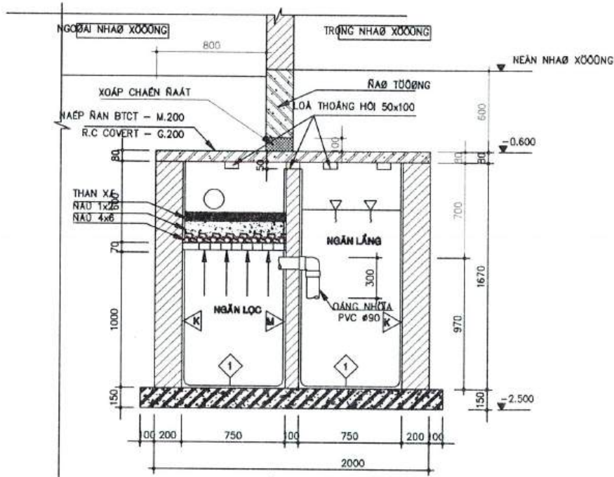
MẶT CẮT SECTION
