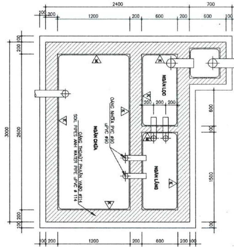
VỊ TRÍ HẦM TỰ HỌAI 1a
