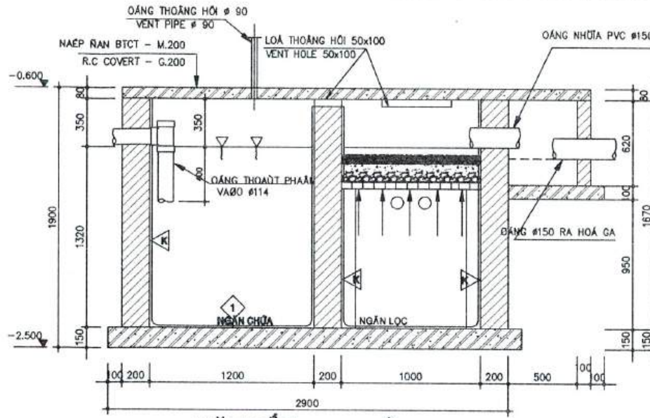
MẶT CẮT SECTION
