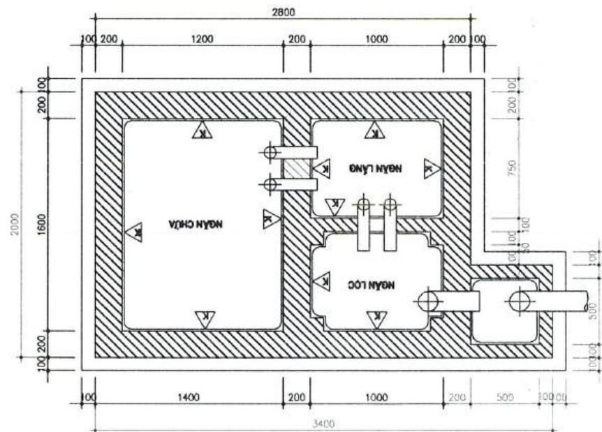
VỊ TRÍ HẦM TỰ HỌAI 2a
