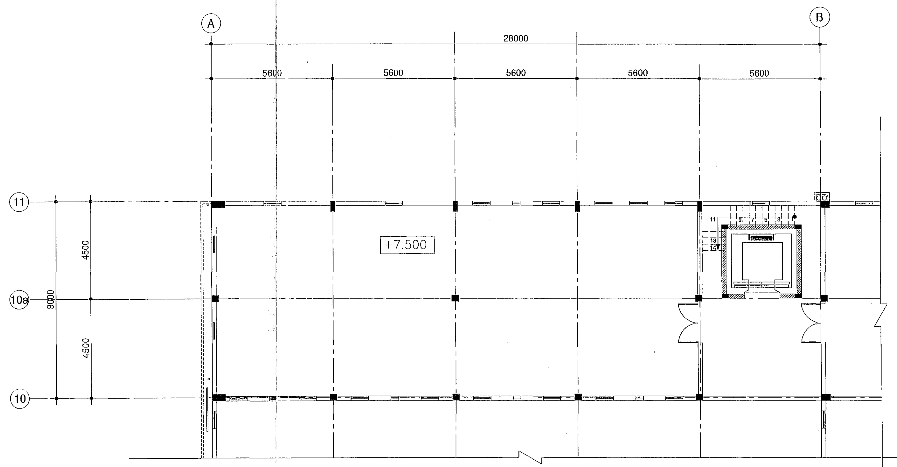
MẶT BẰNG TẦNG 3 (+7.500) 3rd FLOOR PLAN
