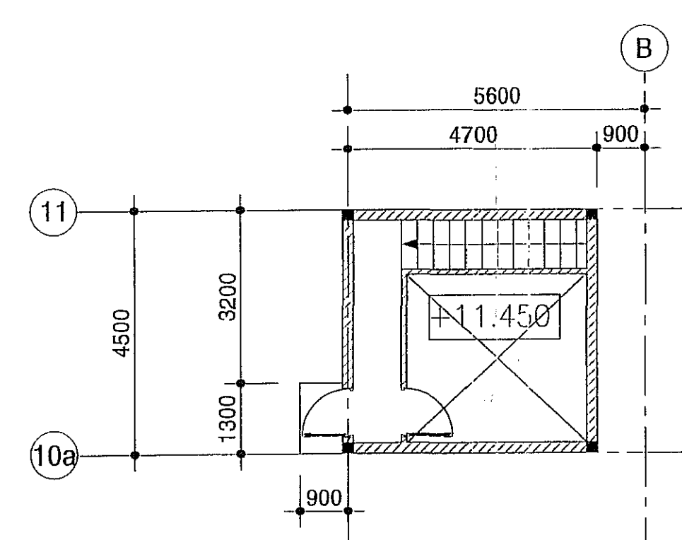
MẶT BẰNG TẦNG KỸ THUẬT THANG MÁY
